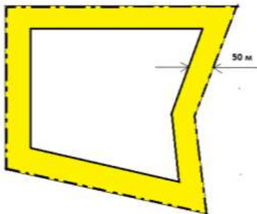
Рис. 15 Опасная зона вокруг границ лесосеки.
